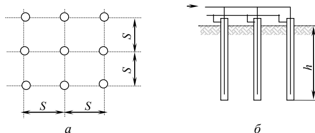
Рис. 1. План (а) і перетин (б) куша з дев'яти теплообмінників
