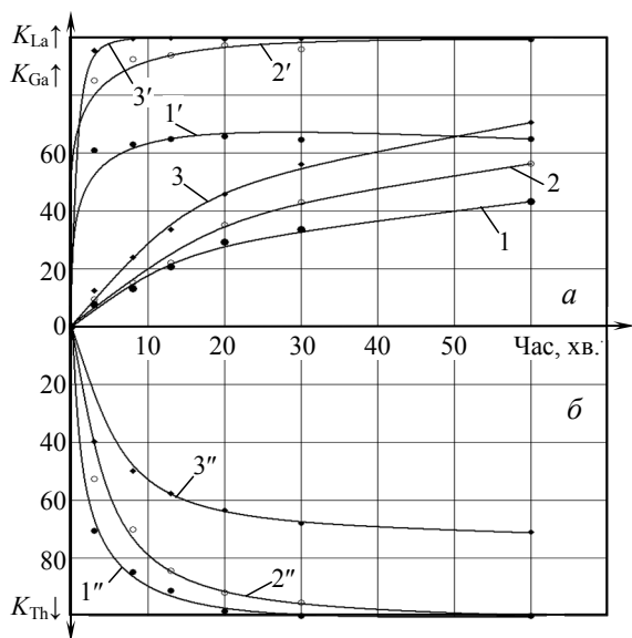
Залежність коефіцієнтів витягу (а) та коефіцієнту осадження (б) від тривалості процесу вилугування для: лангбейніту при n = 80\% (1), при n = 100\% (2), при n = 180\% (3); для галіту при n = 80\% (1'), при n = 100\% (2'), при n = 180\% (3'); для натрій сульфату при n = 80\% (1''), при n = 100\% (2''), при n = 180\% (3'')
