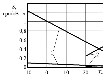
Рис. 3. Зависимость минимальной и максимальной себестоимости S от T_{вх} : 1 — для отопления; 2 — для охлаждения
