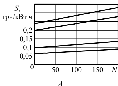
Рис. 1. Зависимость себестоимости S от N : при уровне тепловых потерь, соответствующих нормам (а); при среднем износе трубопровода (б)
