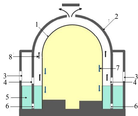
Рис. 4. Система наружного погружения ЗО: 1 — стальная защитная оболочка; 2 — бетонная защитная оболочка; 3 — вход воздуха; 4 — воздушные проемы; 5 — бассейн охлаждения; 6 — водяной проем
