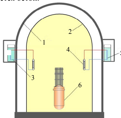
Рис. 11. СПОТ ЗО для проекта ВВЭР-640: 1 — вторичная защитная оболочка; 2 — первичная защитная оболочка; 3 — бак СПОТ; 4 — внутренний конденсатор (теплообменник); 5 — конденсатор; 6 — реактор
