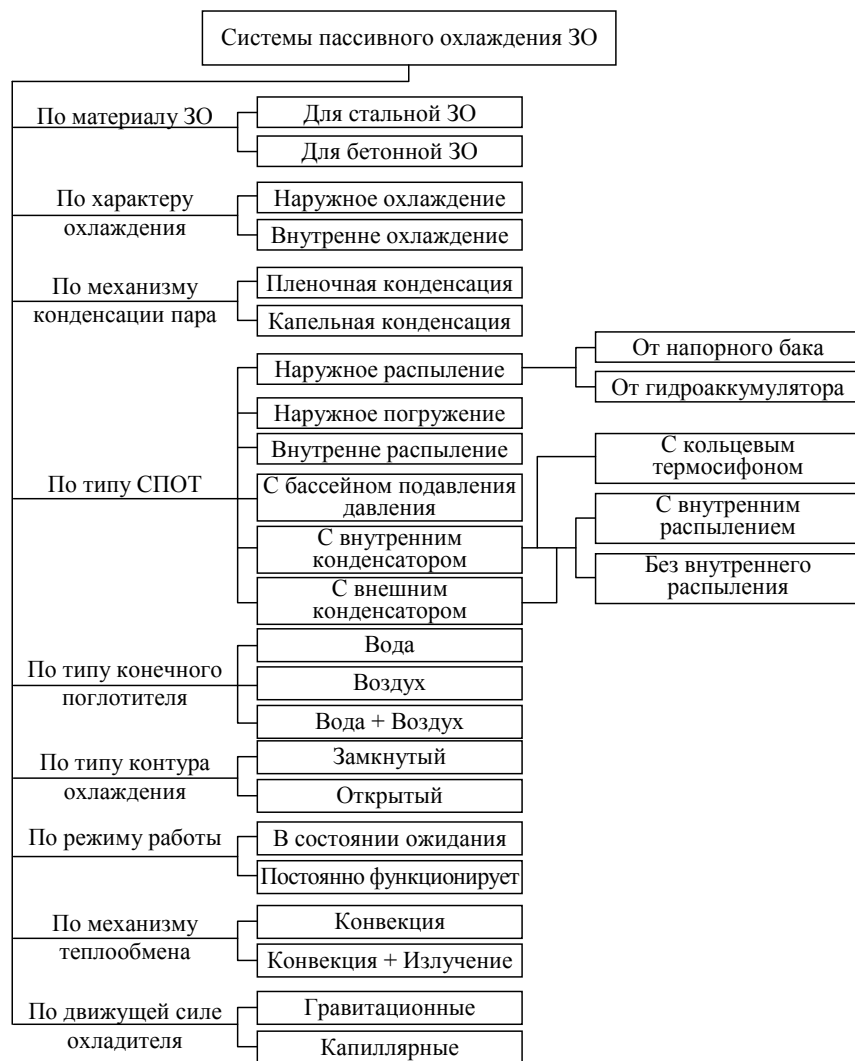
Рис. 1. Иллюстрация классификации СПОТ 3О
