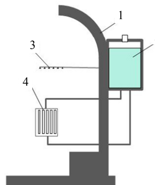
Рис. 9. СПОТ с внутренними конденсаторами (с внутренним распылением): 1 — защитная оболочка; 2 — бассейн; 3 — пассивная распылитель; 4 — внутренний конденсатор
