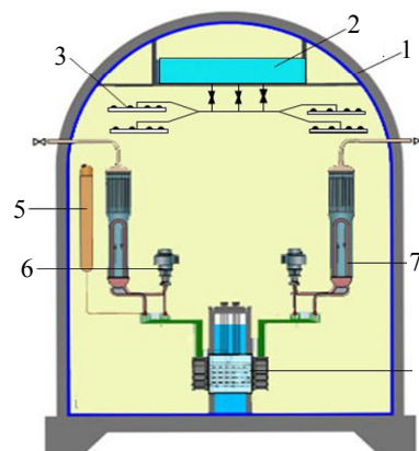
Рис. 5. СПОТ с внутренним распылением проекта ACR-1000: 1 — стальная защитная оболочка; 2 — бассейн охлаждающей воды; 3 — пассивная спринклерная система; 4 — реактор; 5 — конденсатор давления; 6 — главный циркуляционный насос; 7 — парогенератор (ПГ)
