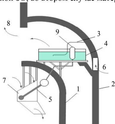
Рис. 10. Система охлаждения с замкнутым контуром охлаждения (с замкнутым термосифоном): 1 — первичная защитная оболочка; 2 — вторичная защитная оболочка; 3 — перегородка; 4 — бассейн; 5 — внутренний конденсатор; 6 — вход воздуха; 7 — металлическая юбка; 8 — выход воздуха; 9 — теплообменник
