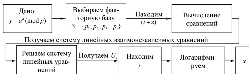
Рис. 1. Схема работы алгоритма исчисления порядка
