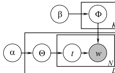
Рис. 2. Графическая вероятностная модель LDA: w — слово (наблюдаемая переменная); t — тема (скрытая переменная); D — коллекция документов; N — длина документа в словах; K — количество тем в коллекции; \Theta — распределение тем в документе; \Phi — распределение слов в теме; \alpha — априорное распределение Дирихле на параметры \Theta , \beta — априорное распределение Дирихле на параметры \Phi
