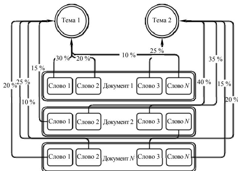
Рис. 3. Модель LDA с выделением двух тем
