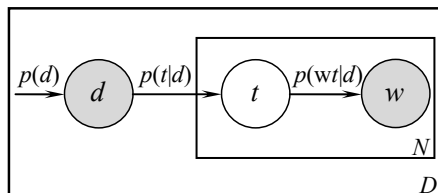
Рис. 1. Графическая вероятностная модель PLSA: d — документ; w — слово; d, w — наблюдаемые переменные; t — тема (скрытая переменная); p(d) — априорное распределение на множестве документов; p(w|t) , p(t|d) — искомые условные распределения; D — коллекция документов; N — длина документа в словах
